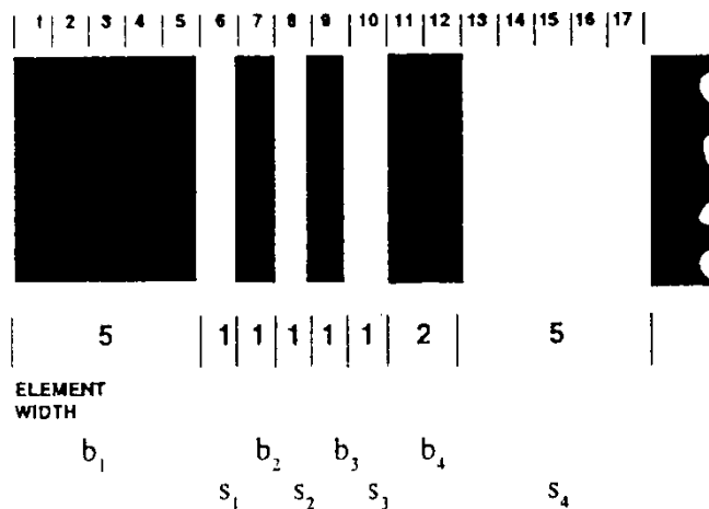
Abbildung 3: Codewort-Symbol
